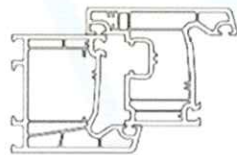
A-A Section
