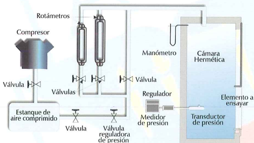
Fig. Nº 1: Esquema montaje experimental
